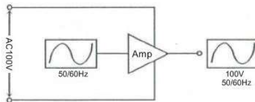
[Active DC Suppression] ブルメスター式（並列）電源ユニット
